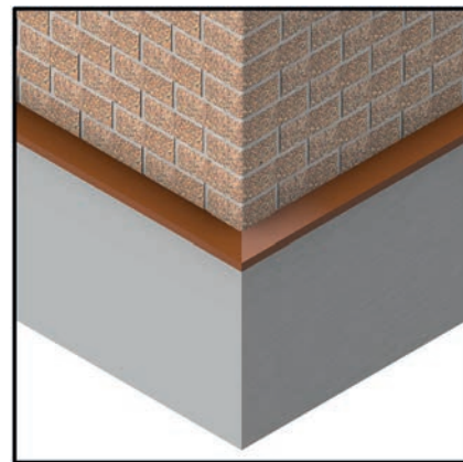
Рис. 22 Устройство внешних углов при помощи угловых элементов.
