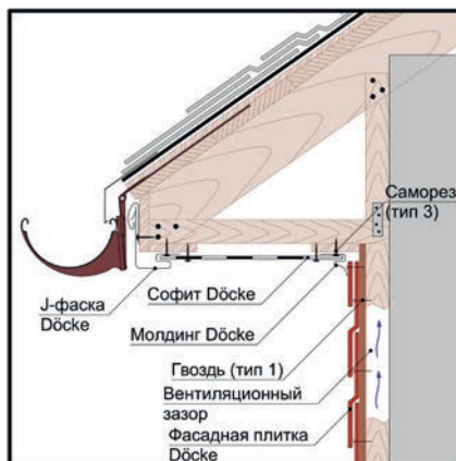
Рис. 33 Примыкание фасадной плитки к карнизному свесу.
