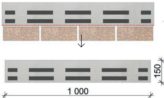
Рис. 7 Изготовление стартовой полосы.
