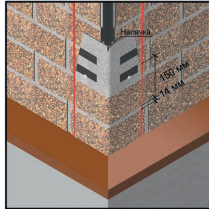
Рис. 21 Монтаж последующих угловых элементов.
