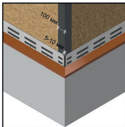
Рис. 8 Крепление металлических отливов.
