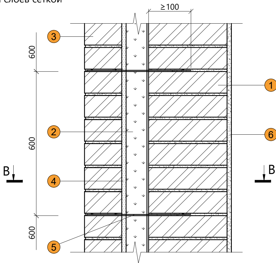
Б - Б
