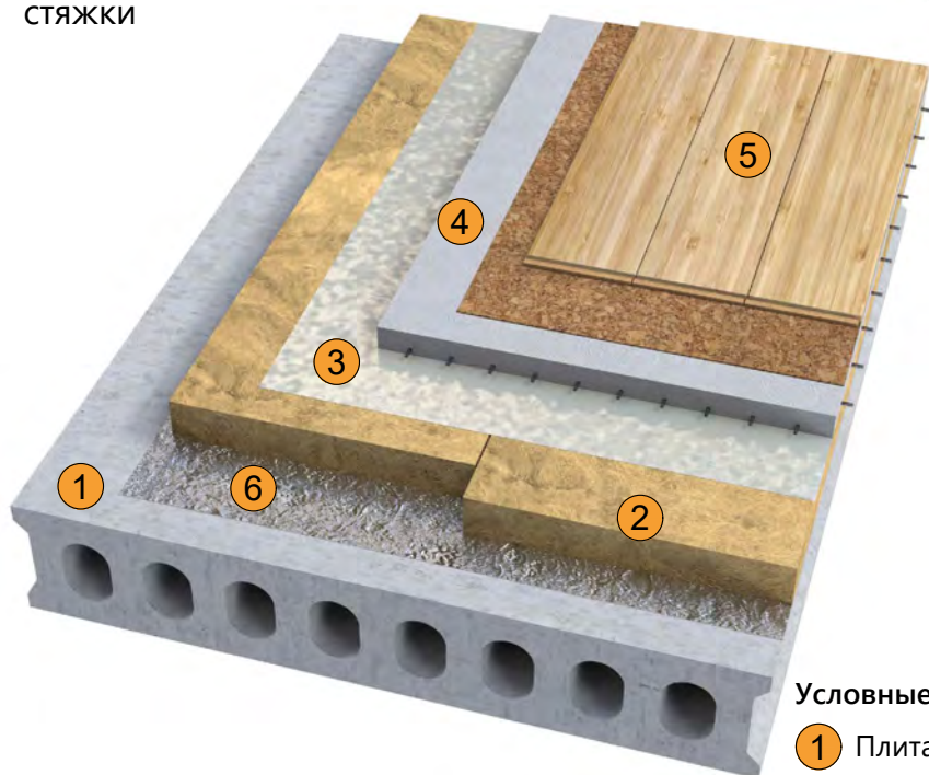
Б. Полы с устройством цементно-песчаной стяжки
