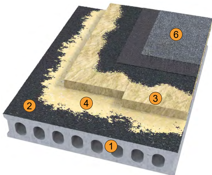
А. Однослойная изоляция
