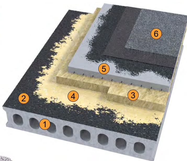
Б. С устройством цементно-песчаной стяжки
