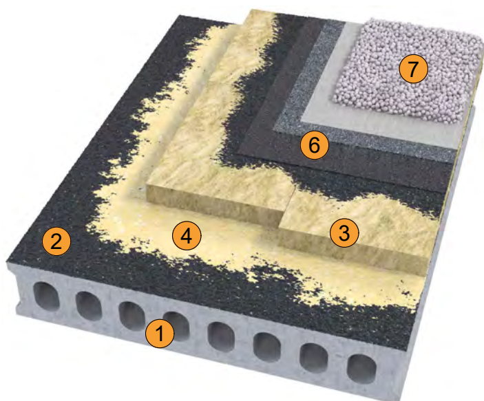
В. С защитным покрытием из гравия
