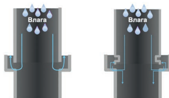
Конструкция соединения без углубления
